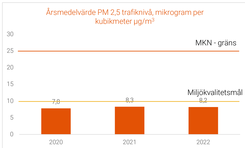
Figur 33 Diagrammet visar årsmedelvärde för halten av små partiklar PM2.5 i luften samt miljökvalitetsnormens gräns och miljökvalitetsmålets riktvärde. Källa: Miljö-och hälsoskydd Luftkvalitetsrapport 2022, Helsingborgs stad
