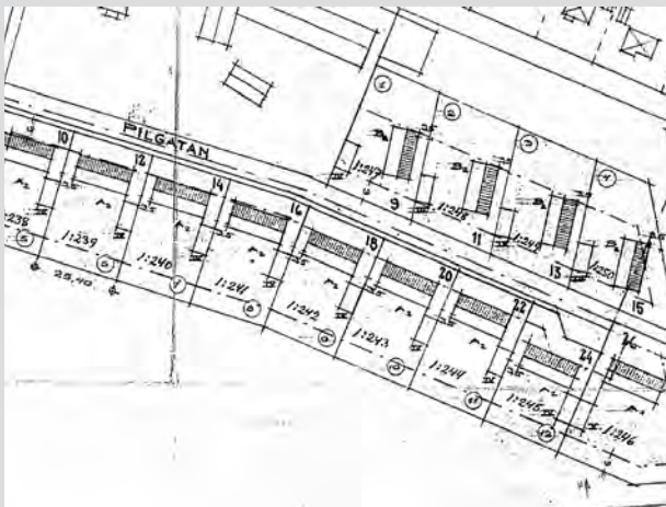
Ursprunglig situationsplan som visar "Marabouhusen" längs Pilgatan.
