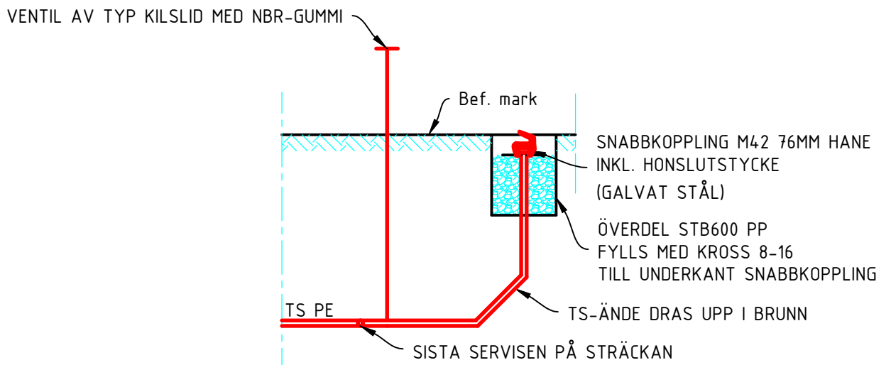
Sektion A-A
