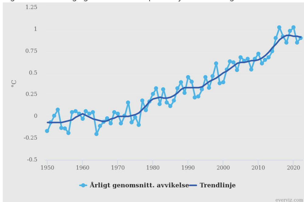
Figur 1. Förändring i global medeltemperatur jämfört med genomsnittet 1950-1980, °C
